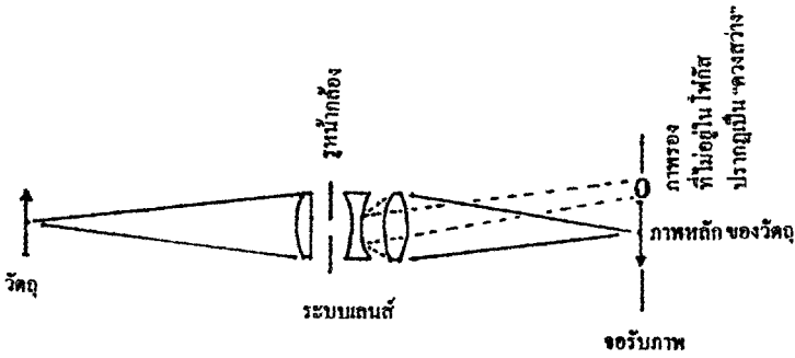
รูป 4 การเกิดภาพจริงที่ไม่อยู่ในโฟกัส จากแสงสะท้อนภายในระบบเลนส์ วาดภาพโดยพรชัย พัชรินทร์ตระกูล แห่งจุฬาลงกรณ์มหาวิทยาลัย
