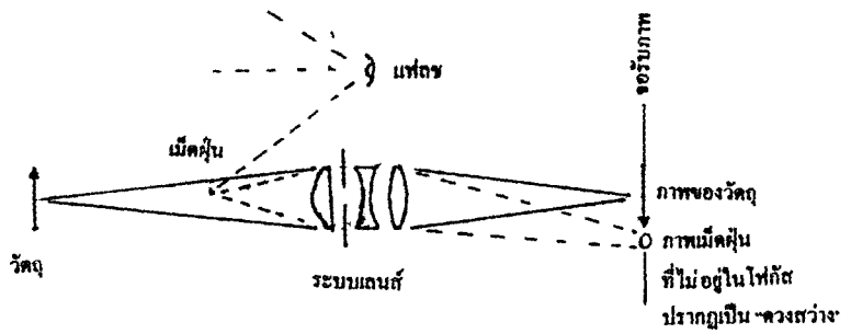
รูป 3 การเกิดภาพเมื่อดูดที่ไม่อยู่ในโฟกัส วาดภาพโดยพรชัย พัชรินทร์ตะนกุล แห่งจุฬาลงกรณ์มหาวิทยาลัย
