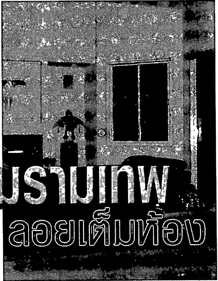
รูปที่ 1 “จตุคามรามเทพ” ลอยเต็มห้อง ดวงกลมส่วนใหญ่นี้ภาพเปิดฟังก์ชันที่ไม่อยู่ในโฟกัส ถ่ายภาพโดยแกรี ชวาทซ์ และแคเธอรีน คริส #ห้องมหาวชิราวุธไฮอริโซนา
