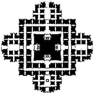
ภาพที่ ๒-๓ : ผังของเจดีย์-วิหาร อานันท แกนทึบสี่เหลี่ยม ตรงกลางเป็นระบบเสากลางรับน้ำหนัก ซึ่งเว้ากลางที่ด้าน ทั้งสี่ เพื่อประดิษฐานพระพุทธรูปด้านละองค์ และมีมุขยื่น ออกมาเท่ากันทั้ง ๔ ด้าน
